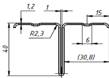
Профиль Т-образный
